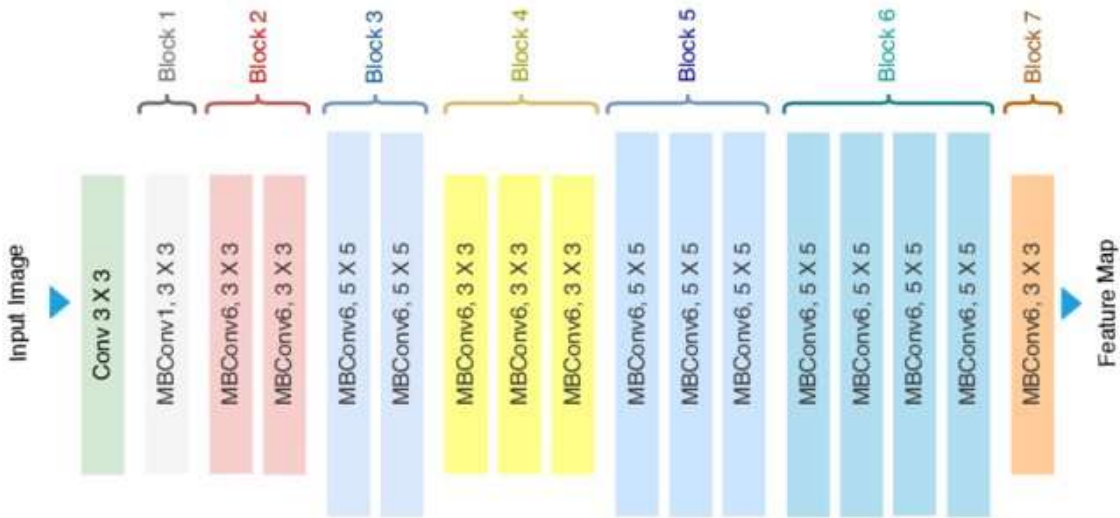
Hình 2: Cấu trúc EfficientNet B0, các biến thể sau này mở rộng từ phiên bản B0 (Ahmed & Sabab, 2021; Tan & Le, 2019). Các mạng EfficientNet thường được huấn luyện trước sử dụng bộ dữ liệu hình ảnh sẵn có. Các tham số của mô hình có thể được sử dụng và được tinh chỉnh (fine-tune) sử dụng EuroSat hoặc các bộ dữ liệu khác
